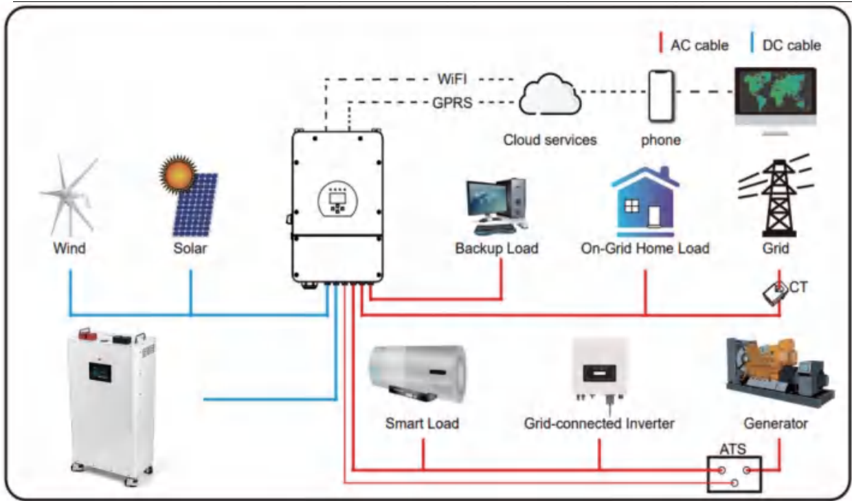
系统连接图System Connection Diagram
