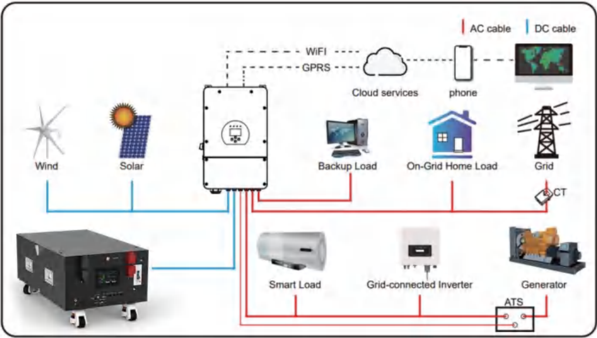
系统连接图System Connection Diagram
